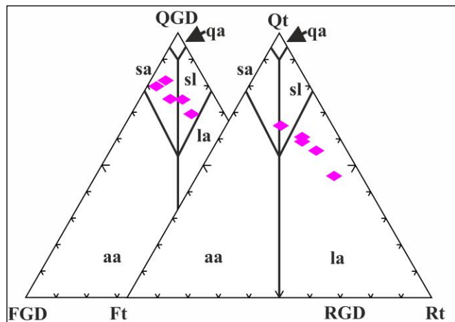
3. ábra – A Jakabhegyi Formáció kimérési eredményei (Pettijohn et al., 1973 alapján), ahol GD és t a kimérési eljárásokat jelentik, qa – kvarcarenit, sa – szubarkóza, sl – szublitenit, aa – arkóza, la – litarenit
