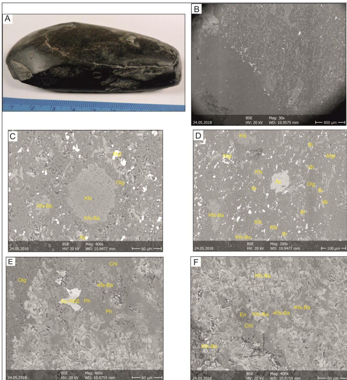
1. ábra – A 74.44.5 leltári számú kőeszköz makroszkópos és BSE-felvételei. A: Makroszkópos kép; B: Átnézeti BSE-kép; C: Káliföldpát Ba-mentes maggal és Ba-dús szegéllyel; D: Ba-dús és Ba-mentes káliföldpátszemcsék; E: Ritkaföldfém-tartalmú epidot; F: Relikt ensztatitszemce a mintában
