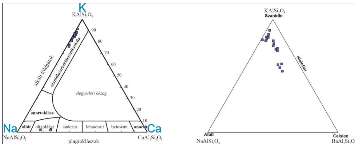
3. ábra – Földpátok ásványkémiái elemzése az Or-Ab-An és az albit-sanidin-celsian háromszögdiagramokban
