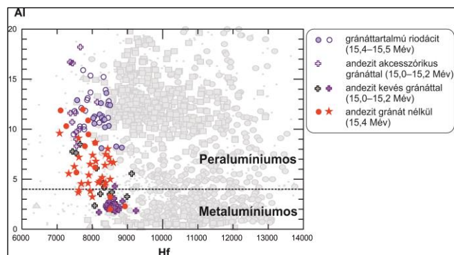
1. ábra – A Visegrádi-hegységben vizsgált kőzetekben előforduló cirkon kristályok Al- és Hf-tartalma (ppm) Peralumínios / Metalumínios határvonal: Trail és munkatársai (2017) alapján. A háttérben szereplő szimbólumok: szürke négyzet: Új-Zéland, szürke kör: Andok, szürke háromszög: Aleuti-szigetek (GEOROC adatbázis)
