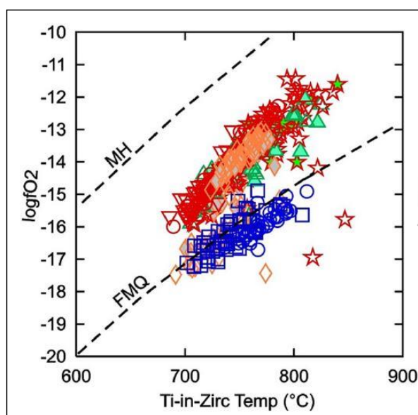
2. ábra – A cirkon kristályok összetételéből számolt hőmérséklet és oxigén-fugacitás értékek eltérő magma típust jeleznek 2 millió évvel korábbi és az utáni időszakban. Felső trend: Piliske és Csomád, alsó trend: Piliske és Kakukk-hegy cirkon kristályai
