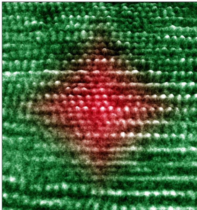
1. ábra – Diafit (kristálytanilag összenőtt gyémánt-grafit) szerkezet a Canyon Diablo meteoritból. A piros gyémánt szimbólummal körvonalazott központi rész (~1,5 nm) jelöli a nanokristályos köbös gyémántot, a zöld szín pedig a grafitot. A piros és a zöld közötti átmeneti szín a gyémánt és grafit átmeneti kötéstípusára utal
