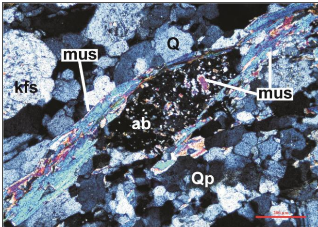
8. ábra – Relikt muszkovit-zárványokat tartalmazó albit, amelyet újonnan képződött muszkovit-kristályok „csomagolnak be” (kereszttezett nikolok, a skála nagysága 200 µm) Rövidítések: ab : albit, kfs : káliföldpát, mus : muszkovit, Q : monokristályos kvarc, Qp : polikristályos kvarc.
