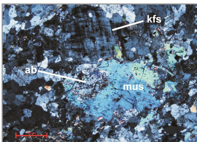
4. ábra – Mikroklinesedő kálföldpát, albitosodó muszkovit (keresztezett nikolok, a skála nagysága 500 μm) Rövidítések: ab : albit, kfs : kálföldpát, mus : muszkovit.
