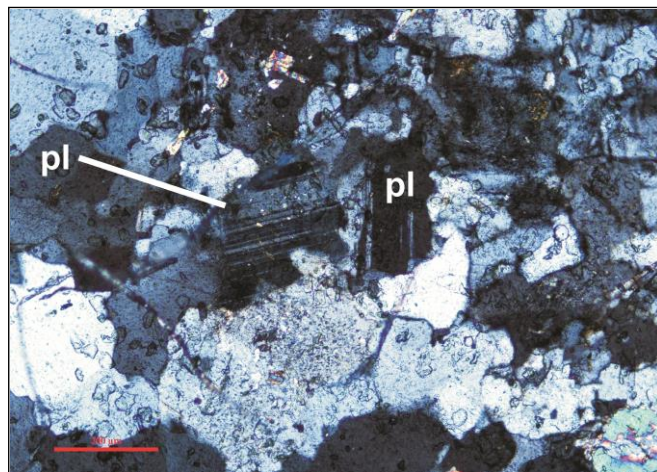
5. ábra – Plagioklászok (keresztezett nikolok, a skála nagysága 200 μm) Rövidítések: pl : plagioklász.
