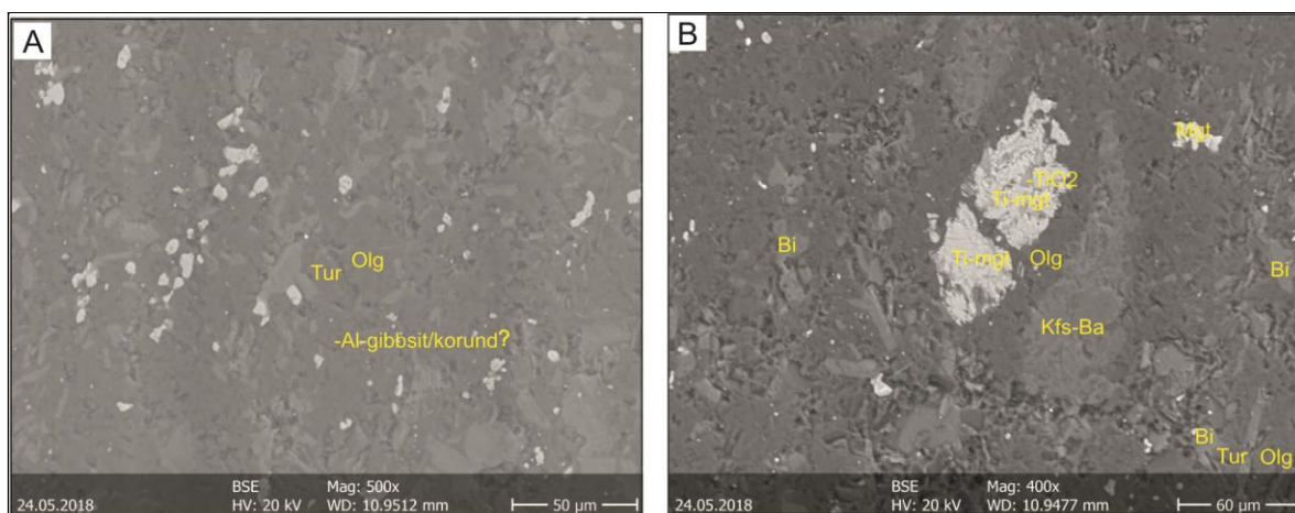
2. ábra – A: Turmalin a 74.44.5 leltári számú kőeszközben; B: Titanomagnetitben \text{TiO}_2 -fázis (rutil?)
