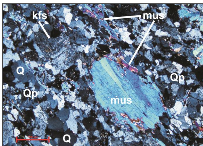
2. ábra – Kőzetszövet: mono- és polikristályos kvarc, földpátok, relik és újonnan képződött muszkovit (keresztezett nikolok, a skála nagysága 500 µm)
