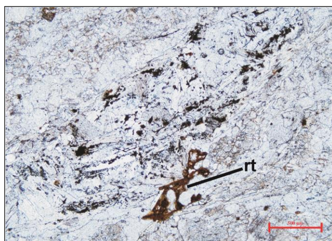
6. ábra – Szagenit-rácsot alkotó rutil-zárvány (1 nikol, a skála nagysága 500 μm) Rövidítések: rt : rutil.
