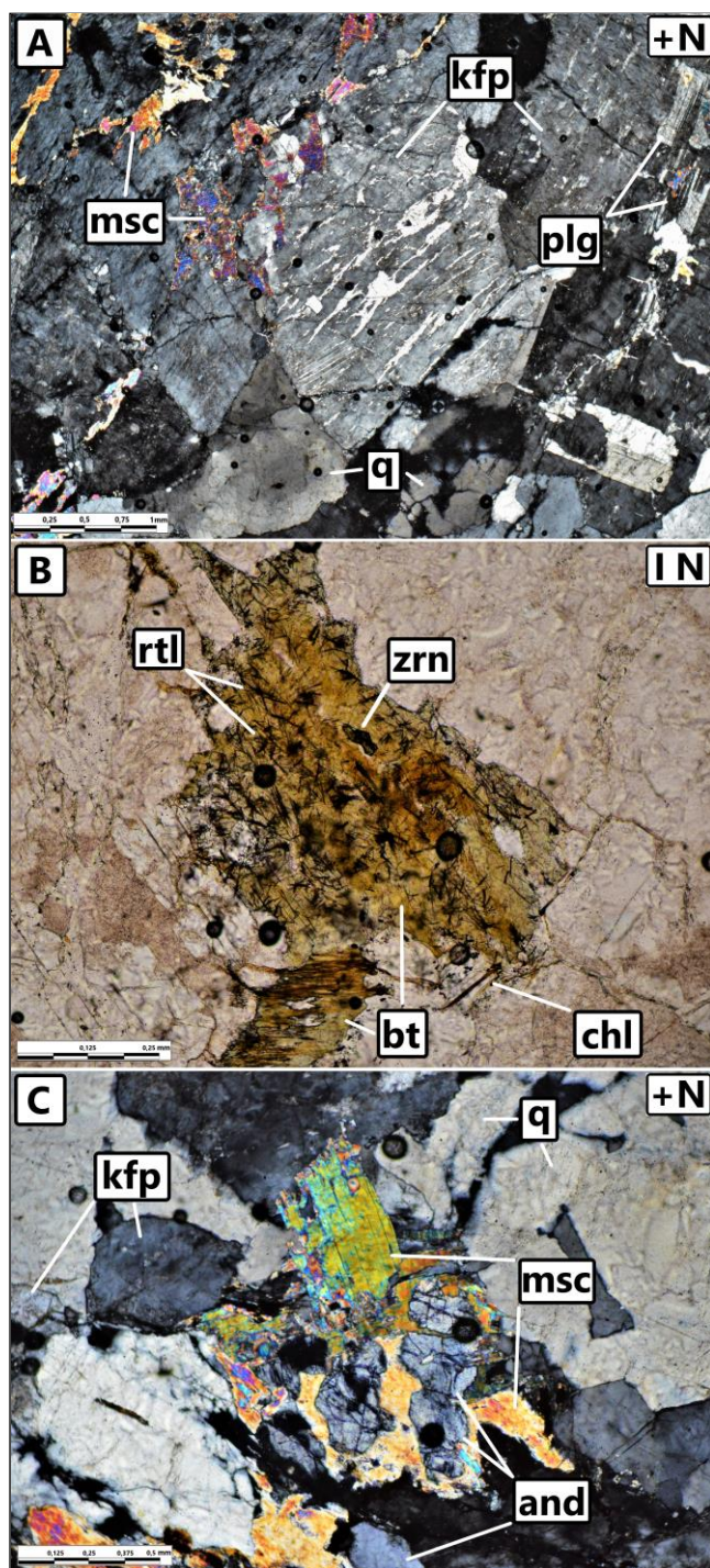
1. ábra – A Nyugat-Mecsek kétcillámú leukogranit kavicsainak polarizációs mikroszkópos felvételei: A) Bükkösd–35 fúrás 167 m: pertites ortoklász, poliszintetikus ikres plagioklász, kvarc és muszkovit; B) Cserdi–14 fúrás 155 m: erőteljesen szételegyedett biotit kristályból kiváló rutiltűk (szagenitrács szerkezet) klorittal és cirkonnal; C) Bükkösd–35 fúrás 167 m: muszkovittal együtt megjelenő andaluzit kristályok Jelmagyarázat: kfp – kálföldpát; plg – plagioklász; q – kvarc; bt – biotit; msc – muszkovit; zrn – cirkon; rtl – rutil; and – andaluzit.
