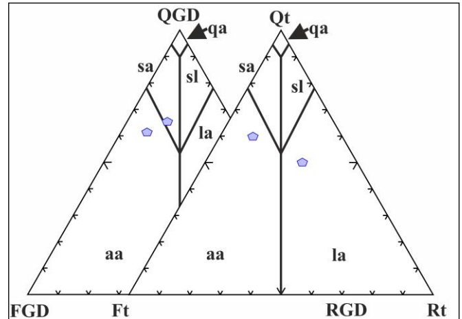
2. ábra – A Kővágószőlősi Formáció kémzési eredményei (Pettijohn et al., 1973 alapján), ahol GD és t a kémzési eljárásokat jelentik, qa – kvarcarenit, sa – szubarkóza, sl – szublitarenit, aa – arkóza, la – litarenit
