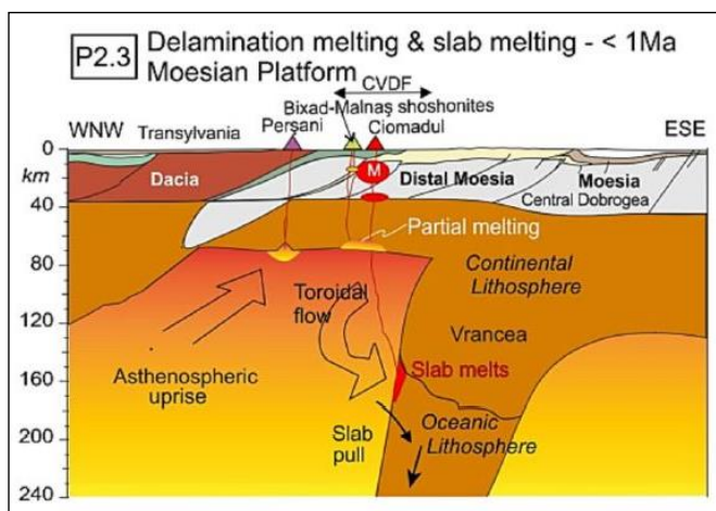
3. ábra – Koncepcionális modell a <1 millió éves vulkáni működés magmaképződésére és geodinamikai kapcsolatára
