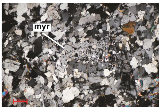
7. ábra – Mirmekit (keresztezett nikolok, a skála nagysága 200 μm) Rövidítések: myr : mirmekit.
