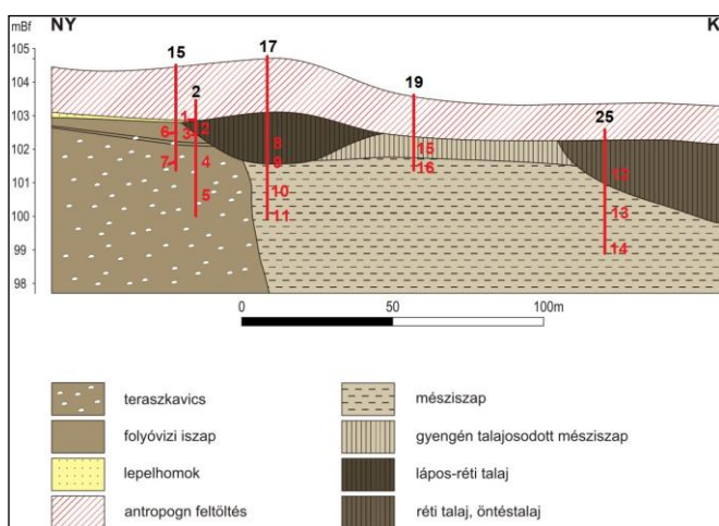
1. ábra – A lelőhely keresztmetszete (Viczián ifj. et al., 2017)
