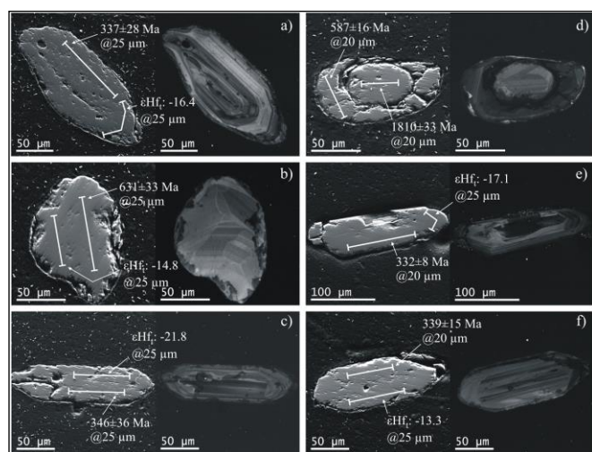
2. ábra – Cirkonok szekunder elektron és katódlumineszcens mikroszkópi felvételei egy ausztriai löszmintából (Stratizing feltárás), U-Pb korokkal és Hf izotóp összetételekkel (a), c), e) és f) Magmás cirkonok oszcillációs zónázottsággal; b) Metamorf kőzetből származó cirkon; d) Átöröklött maggal rendelkező cirkon. Az 1,0 Gévnél fiatalabb korok ^{206}\text{Pb}/^{238}\text{U} korok, míg az 1,0 Gévnél idősebbek ^{207}\text{Pb}/^{206}\text{Pb} korok. A fehér vonalak a lézerablációs „árkok” tengelyét jelölik (átmérőjük a @ jel után mikronban).
