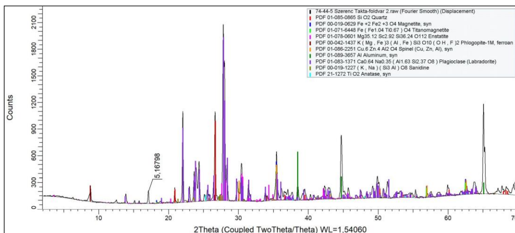
5. ábra – A 74.44.5 leltári számú kőeszköz XRD-felvétele
