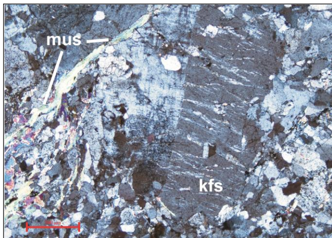
3. ábra – Pertites kálföldpát (magmás eredet), újonnan képződött muszkovit (keresztezett nikolok, a skála nagysága 500 μm) Rövidítések: kfs : kálföldpát, mus : muszkovit.
