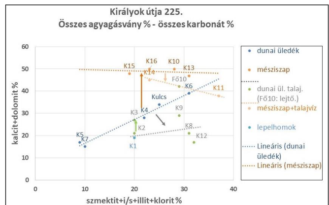
4. ábra – Az összes karbonát az összes agyagásvány függvényében
