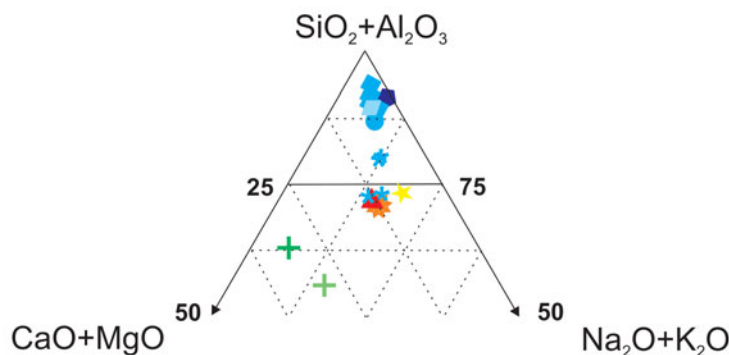
2. ábra – A XI–XIII. századi pásztói üveghuta vizsgált üvegtörődékeinek (saját mérések, Valter, 2015), a diósjenői XIII–XV. századi üveghuta üvegtörődékeinek (H. Gyürky, Miklós, 1992), a történeti alapüvegtípusok átlagösszetételének (Wedepohl és Simon, 2010, Wedepohl et al. 2011), a tári dácittufa teljesközetösszetételének (Zelenka et al., 2004) és kőzetüveg-törődékeinek (Harangi et al., 2005) összetételének összehasonlítása
