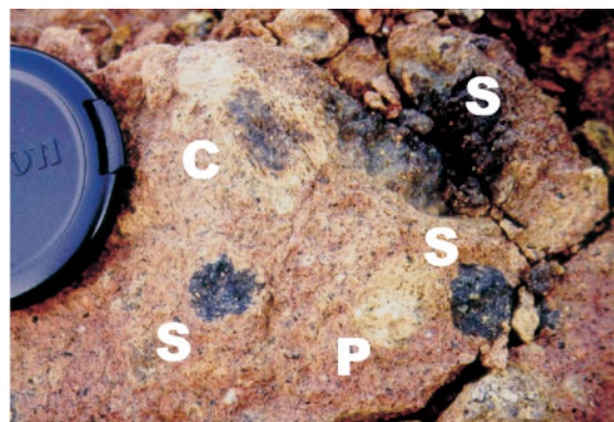
2. ábra – A Bogácsi-egység két fő tagjának terepi megjelenése (Vén-hegy, Bogács): balra fiamme-tartalmú ignimbrit (ÖPE), jobbra: kevert juvenilis törmelékdarabokat tartalmazó piroklaszt-ár kőzete (KPE): S = salak, P = horzsakő, C = összetett salak-horzsakő törmelékdarab
