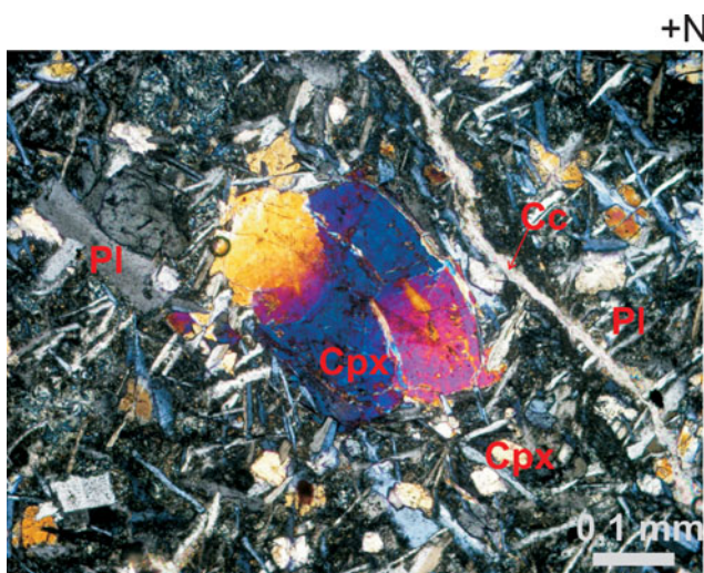
4. ábra – A Szarvaskői Bazalt tipikus szöveti képe polarizációs mikroszkópban (Cc – kalcit, Pl – plagioklász, Cpx – piroxén)
