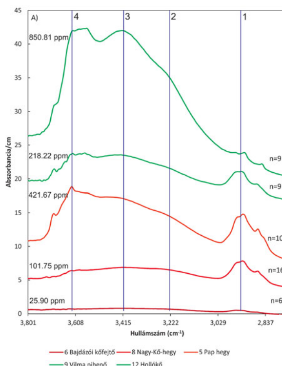
1. ábra – „Nedves” kiértékelés átlagspektrumai 1\text{ cm} -re normálva
