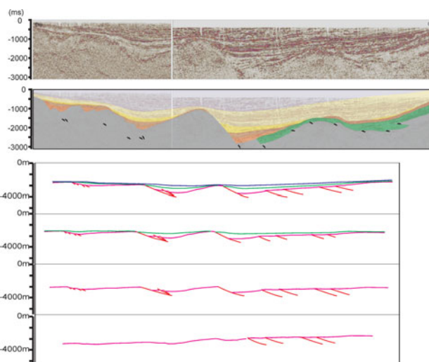
1. ábra – Kisalföldet keresztező Ny-K csapású kompozit szeizmikus szelvény és 2D balansírozása
