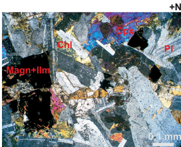
3. ábra – A Tardosi Gabbró tipikus szöveti képe polarizációs mikroszkópban (PI – plagioklász, Chl – klorit, Magn+Ilm – magnetit és ilmenit, Cpx – piroxén)
